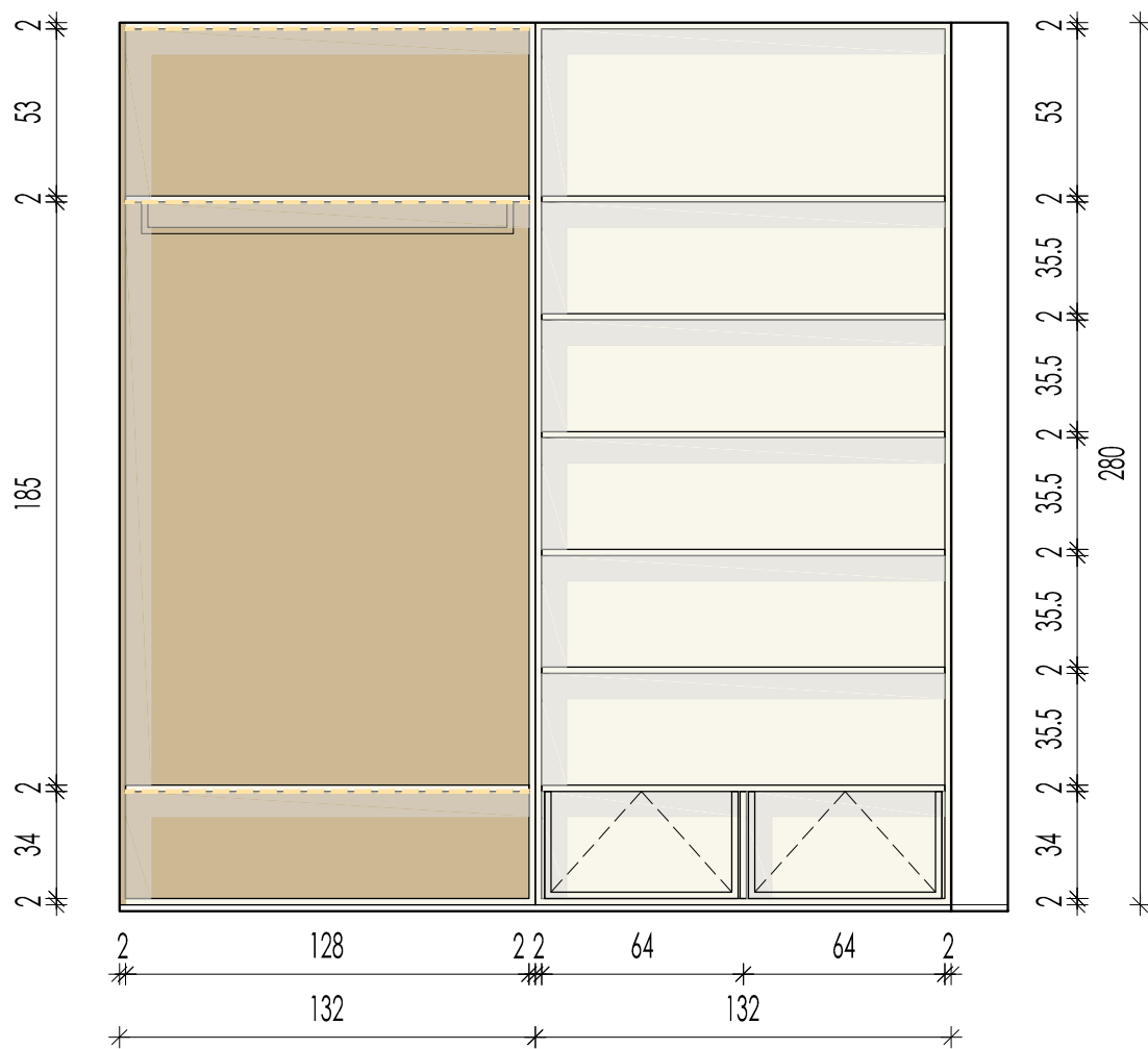
GARDEROBA DZIECI-WIDOK B-B | OTWARTA
