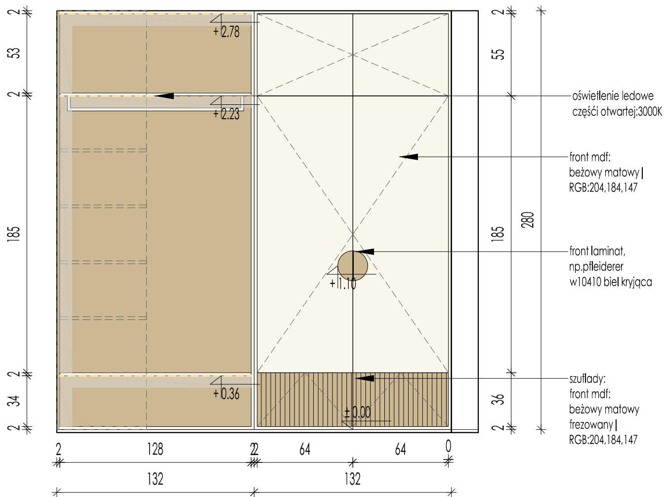
GARDEROBA DZIECI-WIDOK B-B | ZAMKNIĘTA
